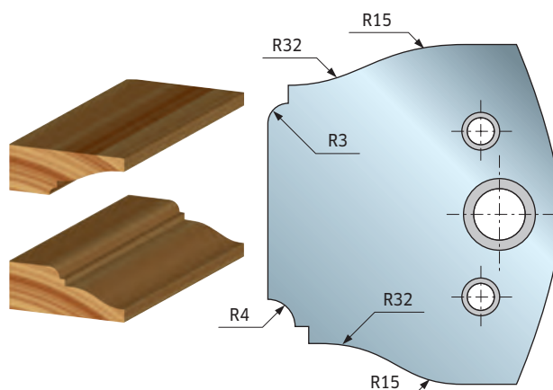
Example of profiled knife - Esempio di coltello profilato
